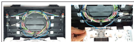
4.2.3 Para el alojamiento del tubo loose de la derivación, puede hacerse manteniendo una reserva o fijándola directamente en la bandeja principal.
