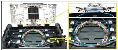
4.1.10 Asegurar los tubos loose de la reserva y de la sangría con las abrazaderas de plástico, y acomode las fibras desnudas del tubo de la sangría en la bandeja principal.
