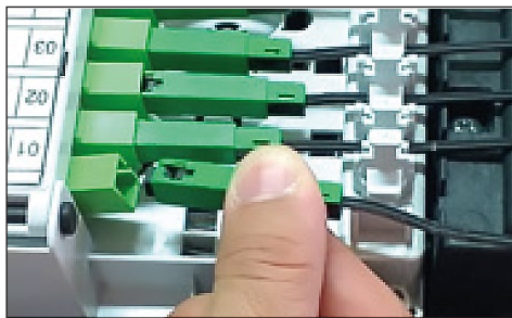
4.4.2 Insertar el drop óptico conectorizado en el adaptador.
