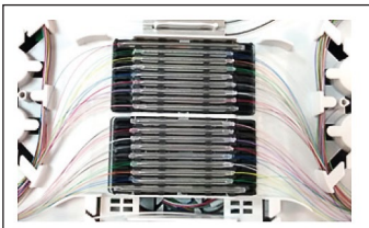
4.2.4 La protección de las fusiones debe realizarse con protectores de empalme de 45 y / o 61 mm de largo (cable de 1,2 mm).
