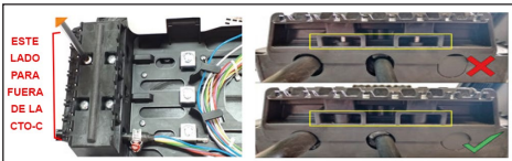
4.3.1. Después de instalar los cables, sean de alimentación o de derivación, monte los bloques de sellado de la entrada de cables y asegúrelos con los tornillos adecuados, apretándolos hasta el final del recorrido.
