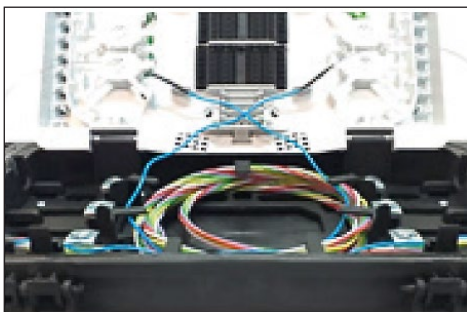
4.1.9 Terminar el tubo loose en el punto de rodillos con cinta de autofusión.
