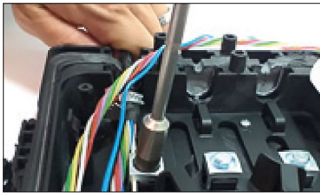
4.1.6 Bloquear el elemento de tracción apretando el tornillo. Cortar el exceso del elemento de tracción del cable.
