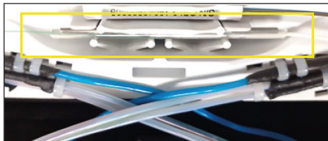
4.1.11 Para la alimentación del splitter de servicio suministrado, hacer la fusión entre el cable "IN" con una fibra de la sangría del cable de alimentación, acomodando la fusión en el alojamiento apropiado.
